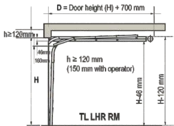
LHR RM – lav takhøydebeslag med dobbel takskinne, bakmonterte fjærer
