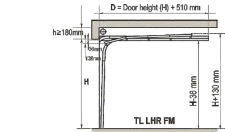
LHR FM – lav takhøydebeslag med dobbel takskinne, frontmonterte fjærer
